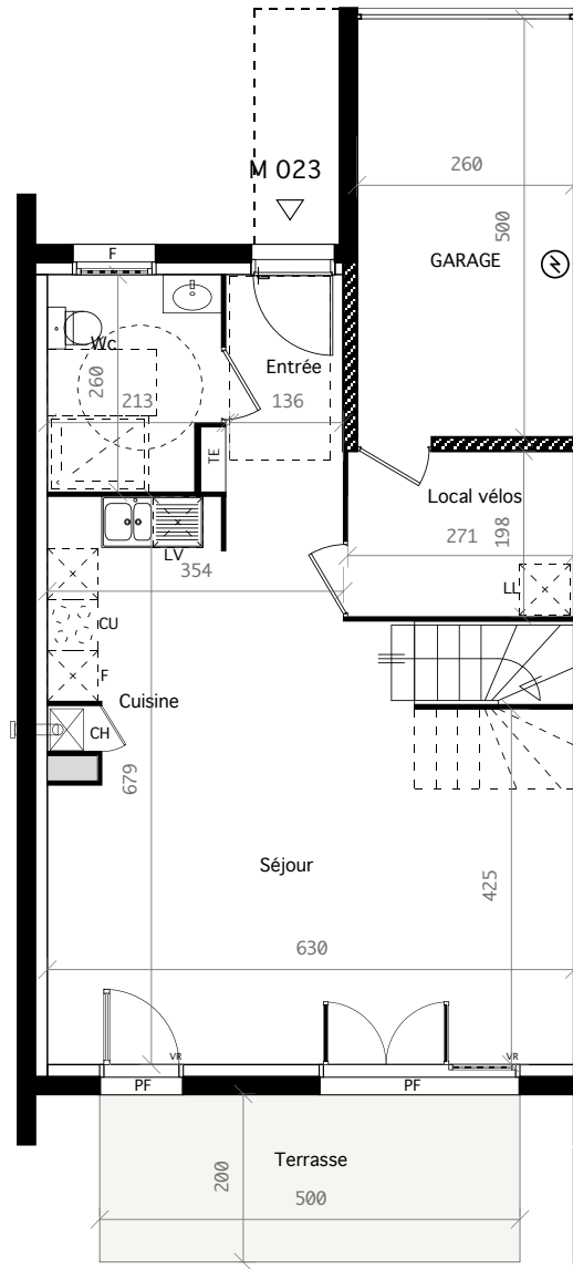
Plan RDC
