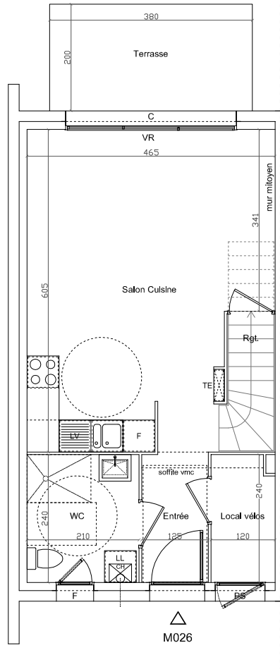
Plan RDC
