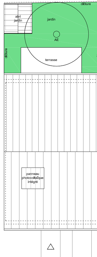
Plan masse
